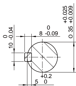
SECTION A-A 1:2
